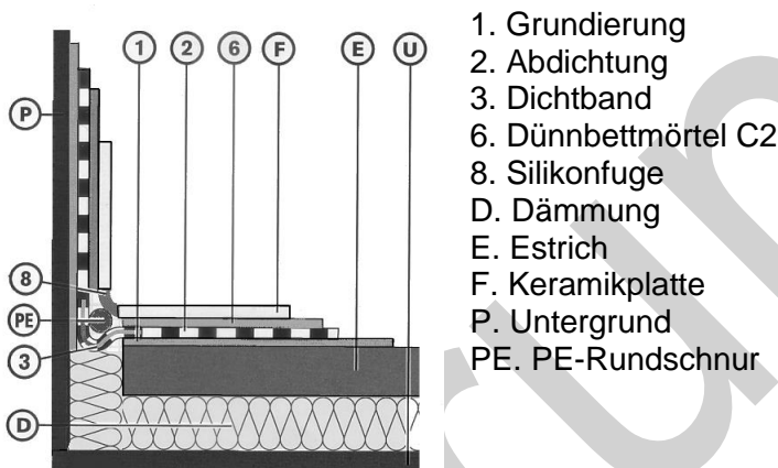
Schematische Skizze
