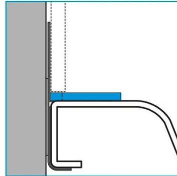
Vertikalschnitt mit Trägerplatte Beim Verlegen von kleinformatigen Platten oder Mosaiken, ist eine Trägerplatte zwingend notwendig.
