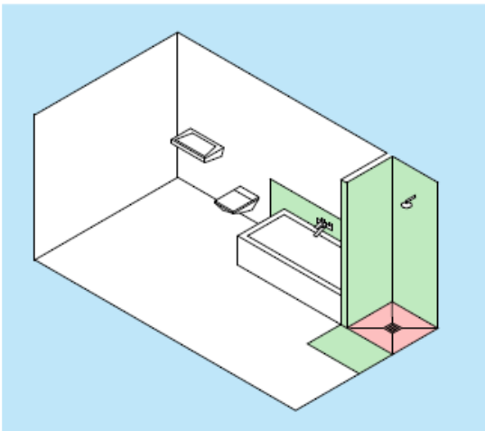
Häusliches Bad mit Badewanne ohne Duschenutzung und planmässig genutztem Bodenablauf im Duschbereich mit Teilbereichsabdichtung vor Dusche auch bei feuchtigkeitsbeständigem Boden
