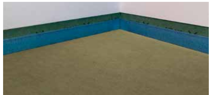
Codex Abdichtung (z.B. Dichtschlämme AX 220) aufbringen inkl. Codex Abdichtungsband BST 150.
